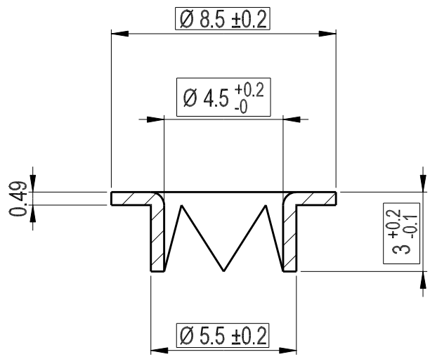
SEZIONE A-A
