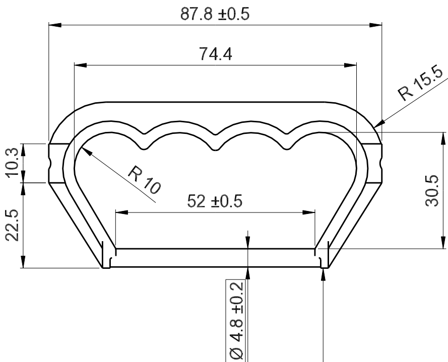
PIEDE DI BLOCCAGGIO DELLA MANIGLIA 0°- 90°
